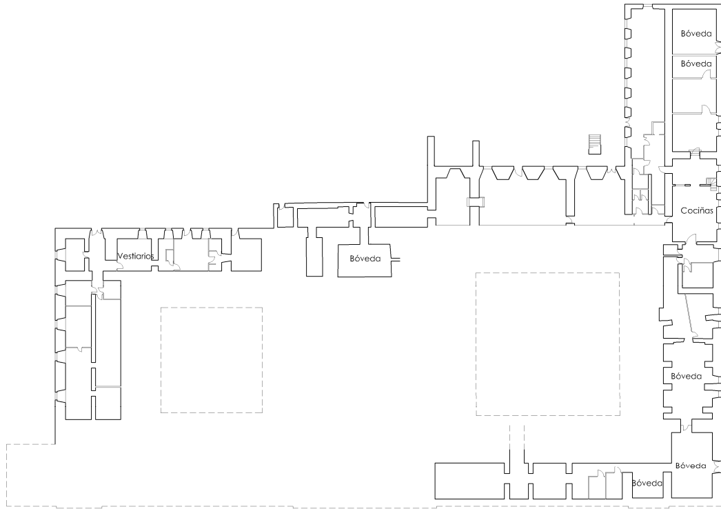
PLANTA SEMISOTO
