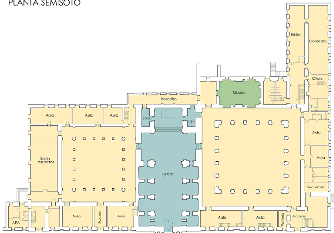
PLANTA BAIXA
