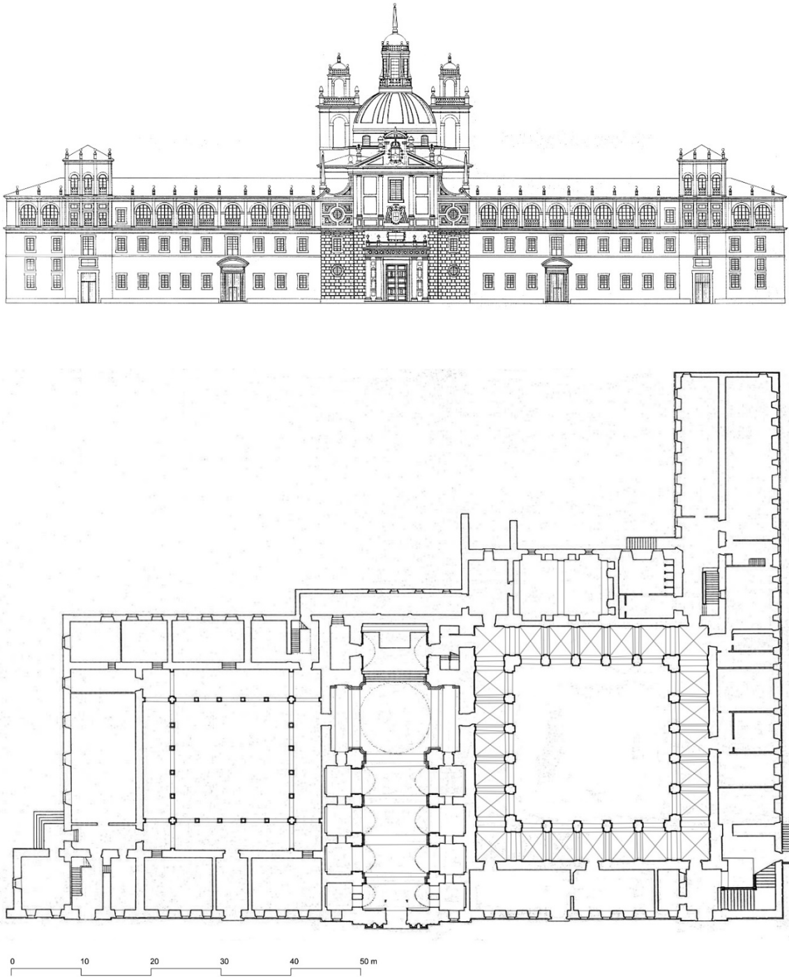
Figura 14. Planta e alzado principal do Colexio de Nosa Señora da Antiga de Monforte de Lemos. Levantamento do arquitecto Carlos Meijide (1984). 34 Escala 1:700. Escala do orixinal 1:200.
