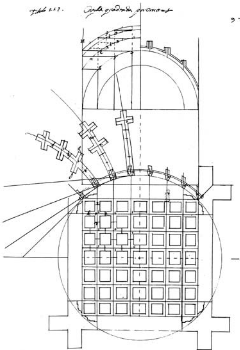
Figura 7 Capilla cuadrada por cruceros en el tratado de Alonso de Vandelvira. En la sección, a la izquierda nervios cuadrados , orientados radialmente. A la derecha, nervios revirados , orientados verticalmente
